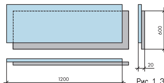
Рис. 1. Элемент пола
